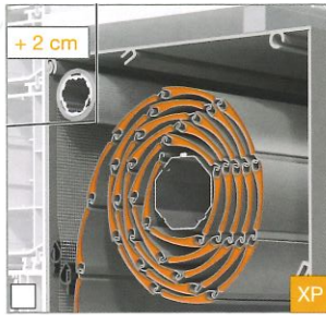
XP-Systeme (Platz für Insektenschutz, Screen, Solar) und P-Systeme.
